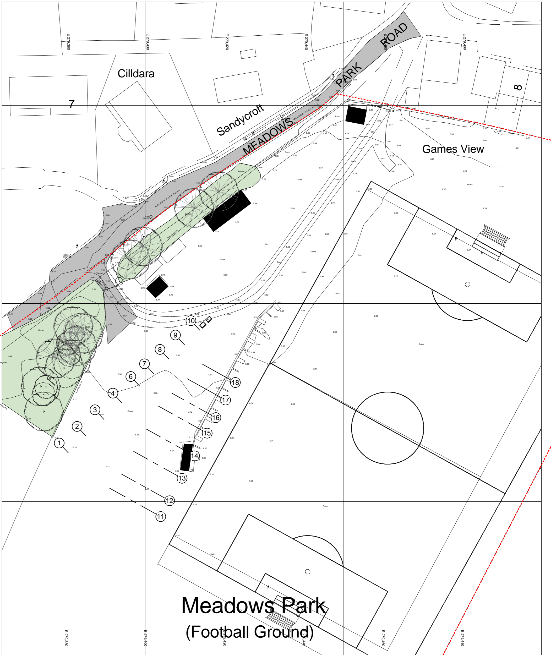
2 Block Plan 2014 1 : 500
